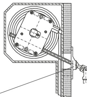
Gelenklager für Kupplungstrichter 23 772.0002 Knick-Kurbel mit Gelenklager und 7 mm 6-kant 23 764.0002 Gelenklager mit Markisenöse 23 731.0002
